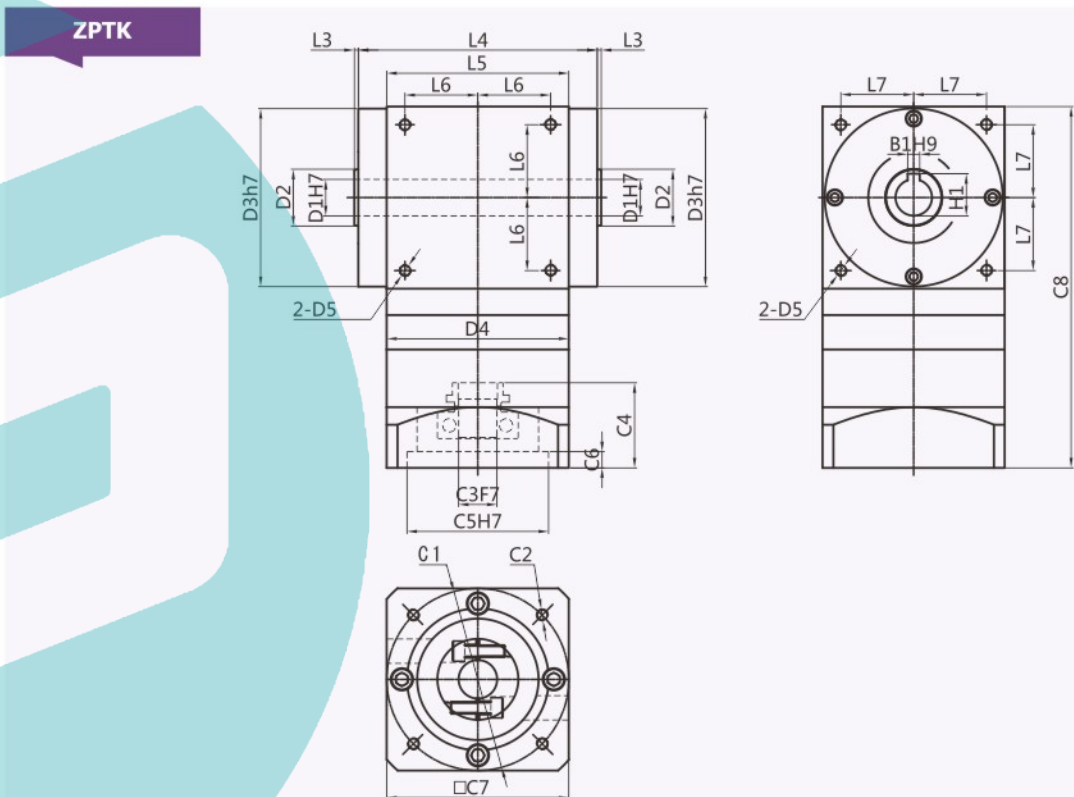
外形尺寸图表 Outline dimensional
