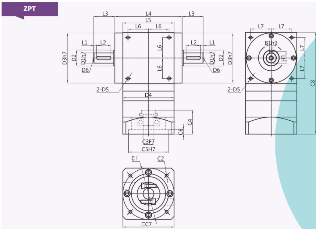
外形尺寸图表 Outline dimensional
