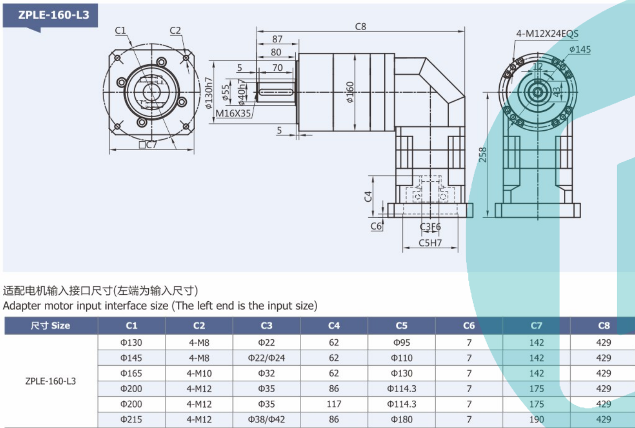
外形尺寸图表 Outline dimensional
