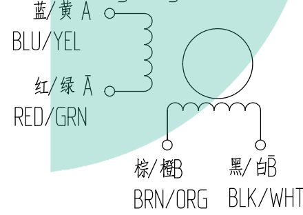
接线图 Wiring diagram:
